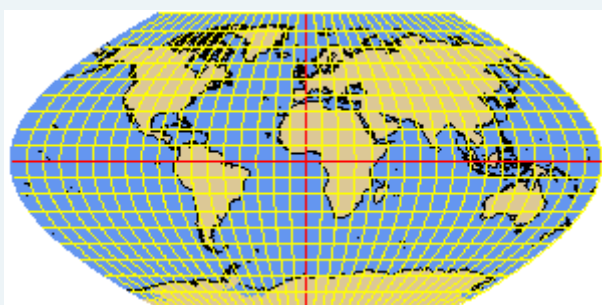
WAGNER3 sinusoidal
