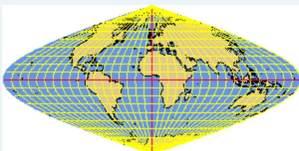
PUTNINS6 hyperbolic
